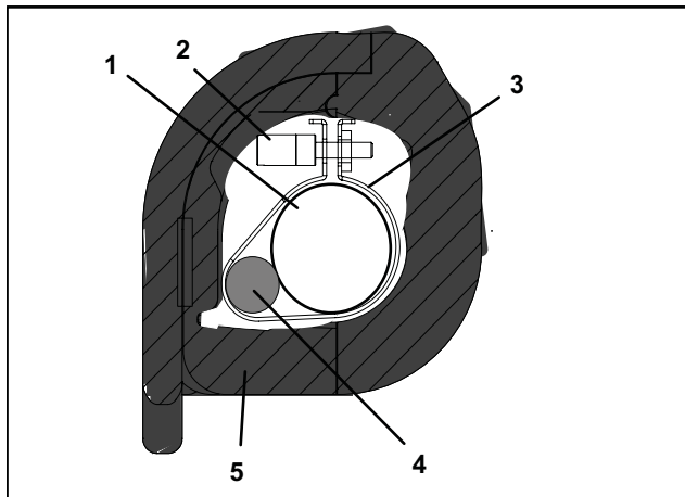
그림 6-19 열팽창 밸브 밸브
