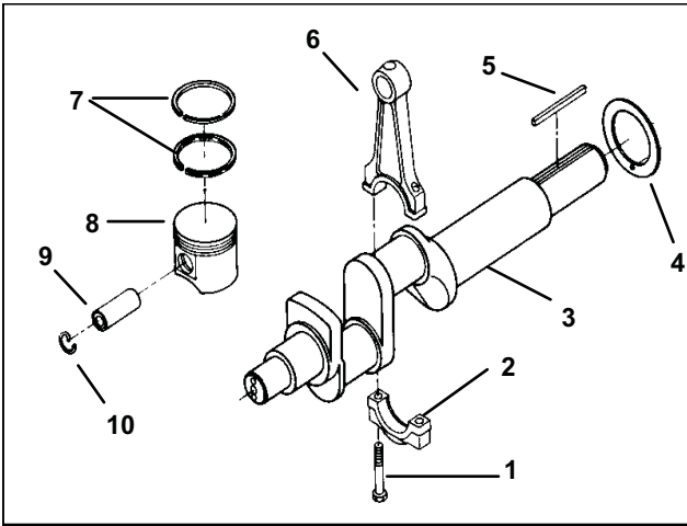
그림 6-13 크랭크축 조립체
