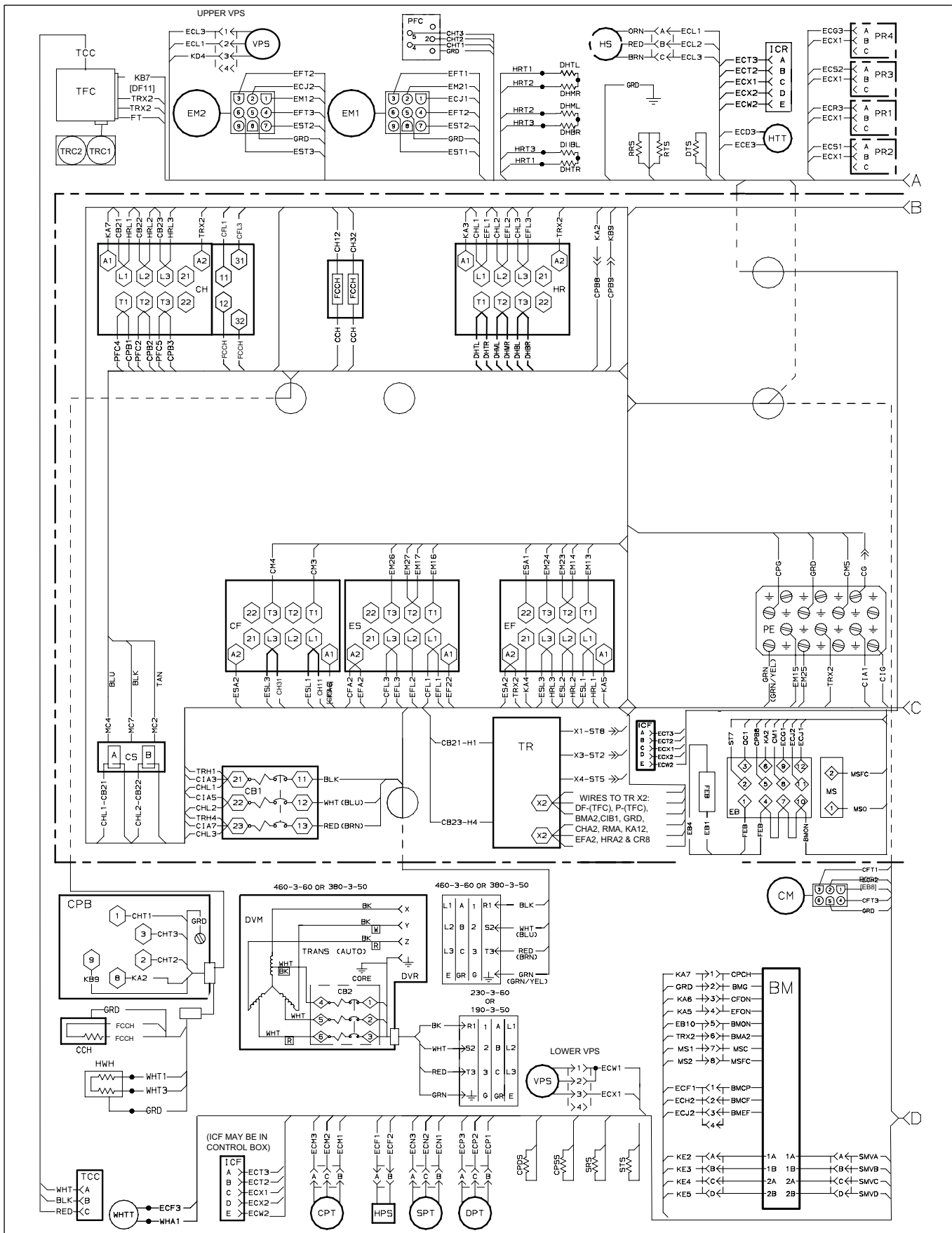
그림 7-7 유닛 배선도 - (1/2)
