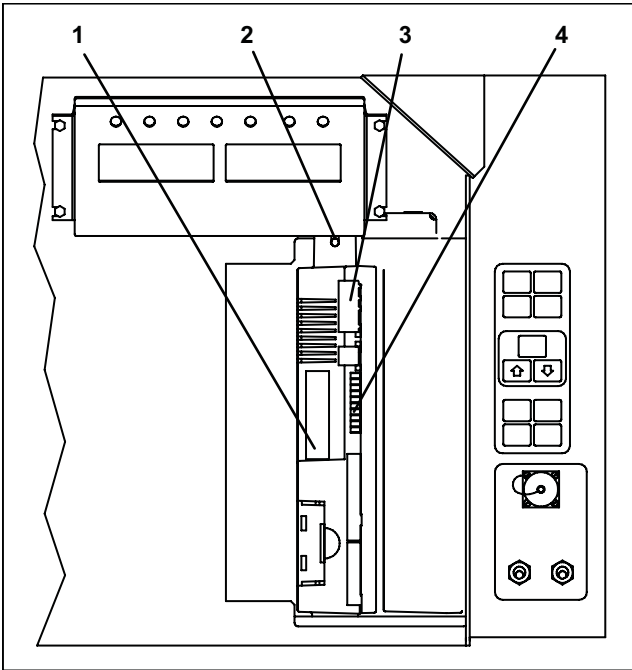
그림 6-26 컨트롤 박스의 컨트롤러 부분
