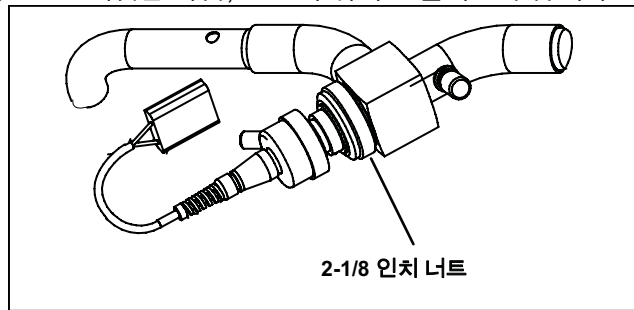
그림 6-24 석션 모듈레이션 밸브 (SMV)
