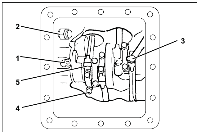
그림 6-8 하단 플레이트 제거
