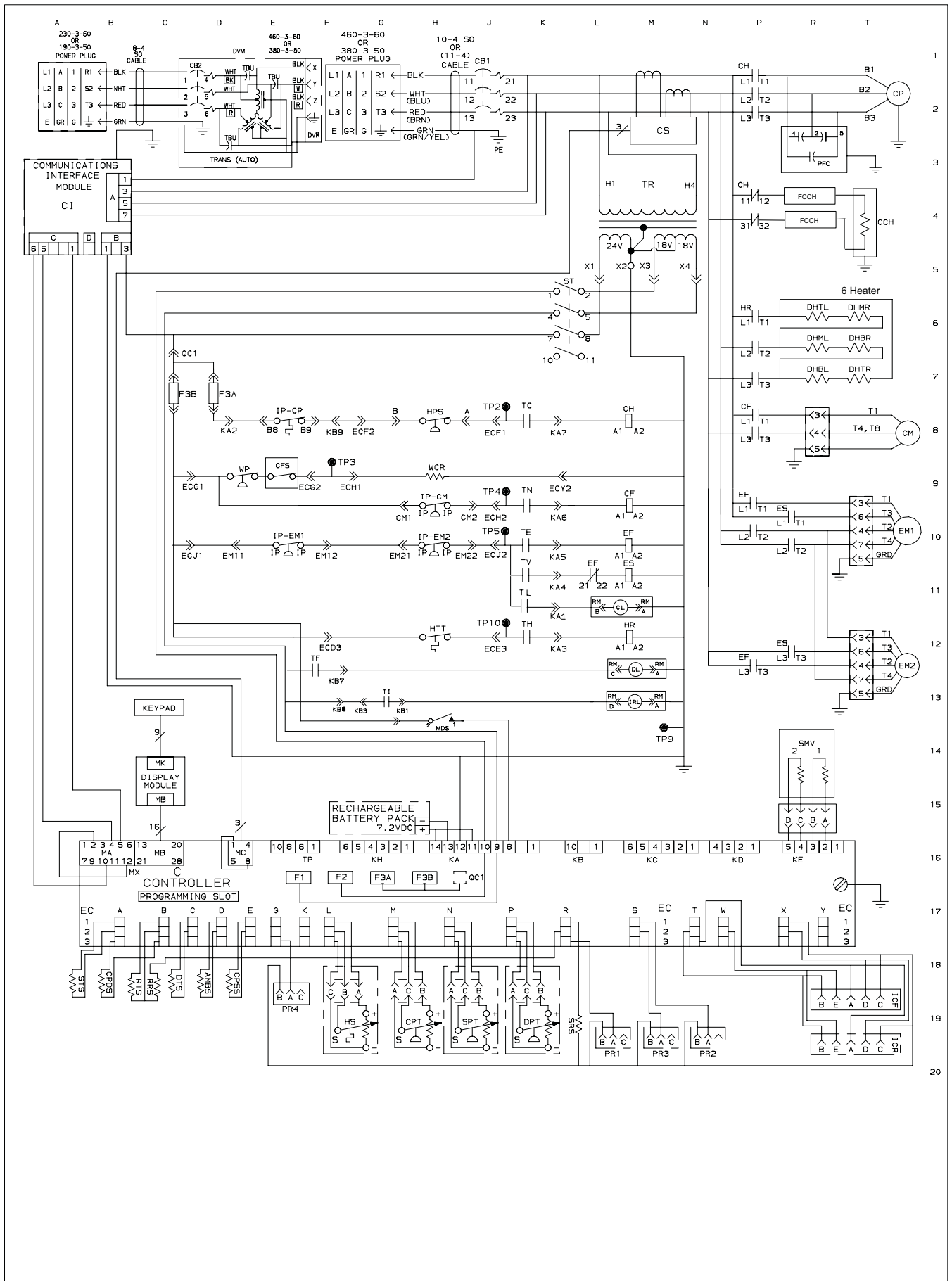
그림 7-2 구성도
