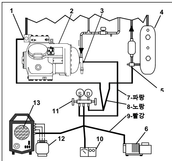
그림 6-4. 냉동 시스템 서비스 연결
