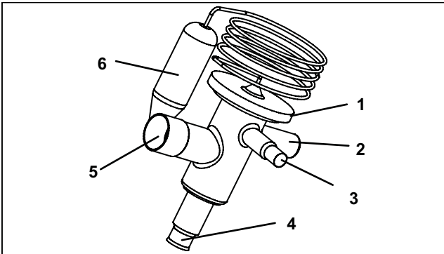
그림 6-20 열 팽창 밸브
