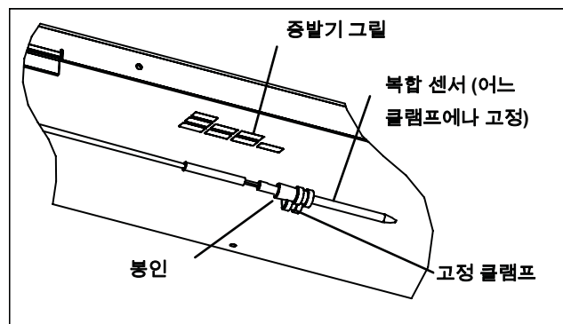
그림 6-30 리턴 센서 위치
