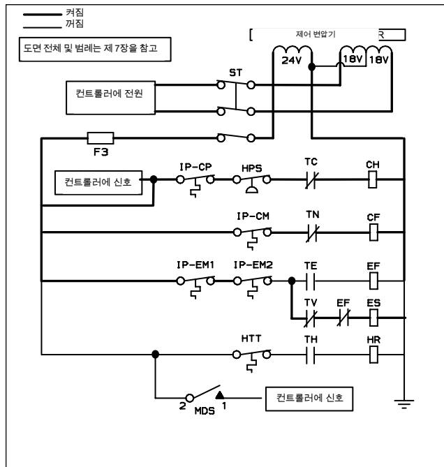
그림 4-7 냉동 모드
