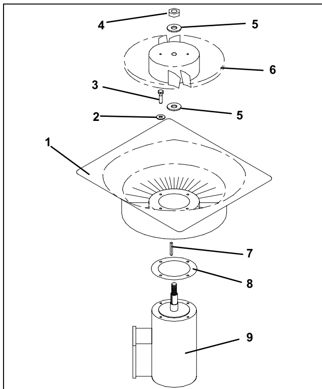
그림 6-23. 증발기 팬 조립체
