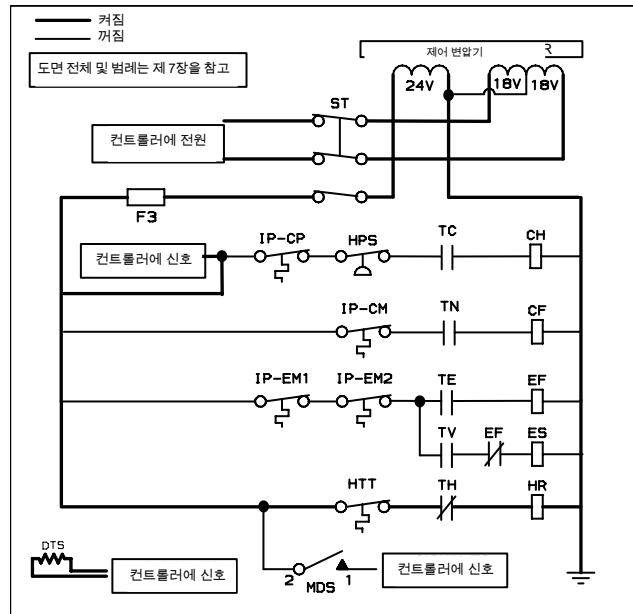
그림 4-8 제상
