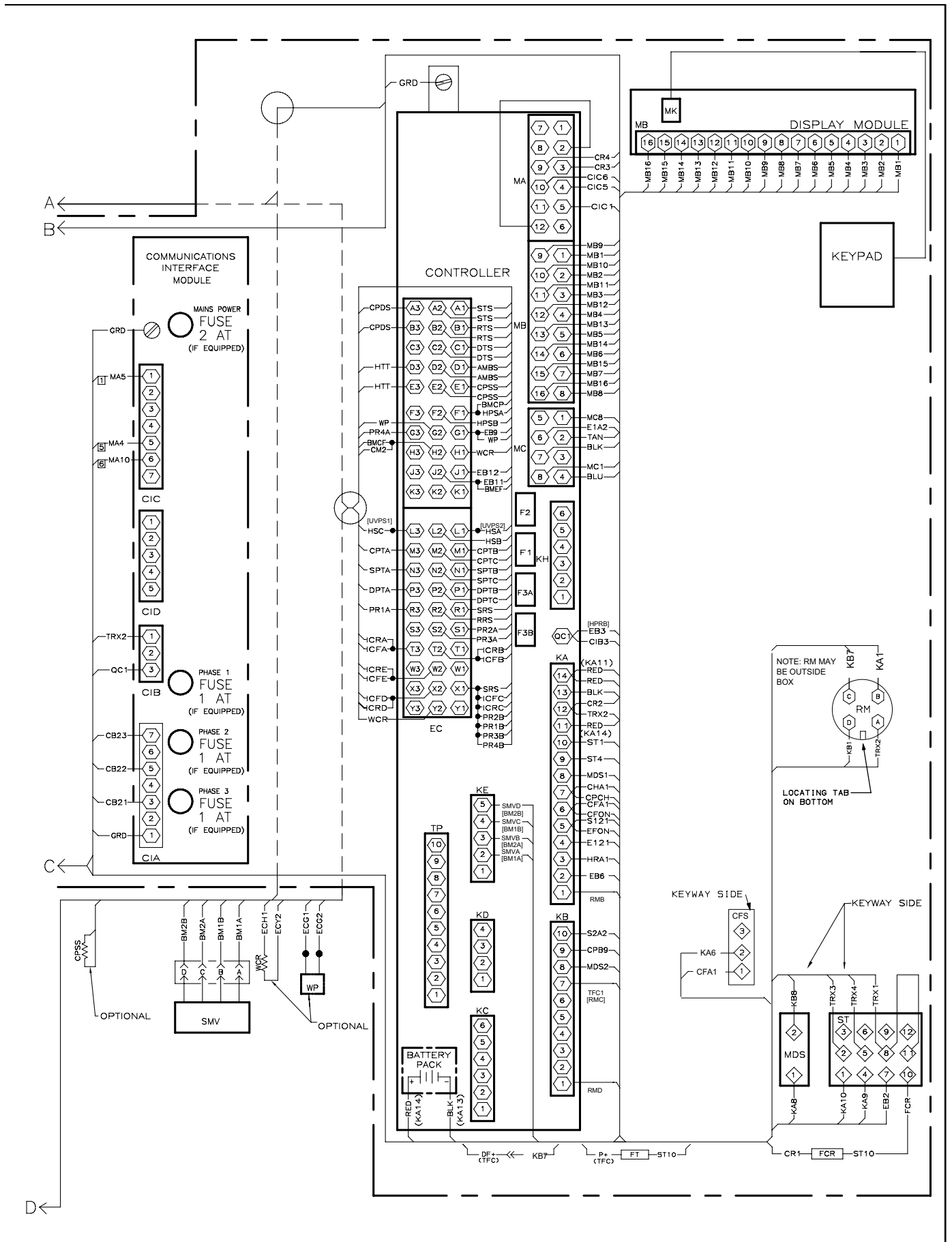
그림 7-8 유닛 배선도 (단일 팬 기능) - (2/2)
