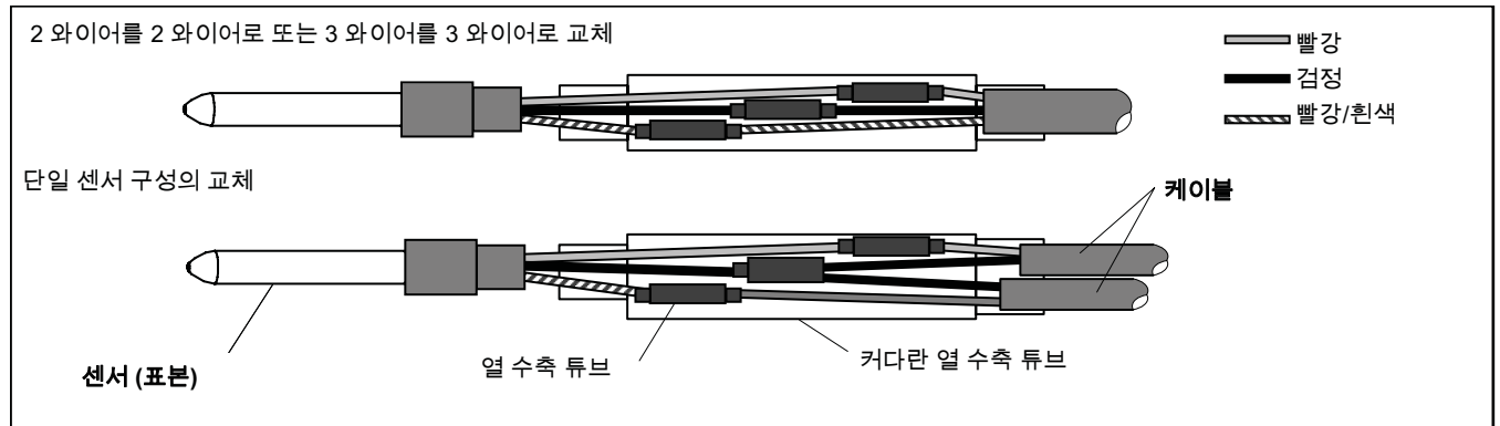
그림 6-28 센서 및 케이블 스폴라이스
