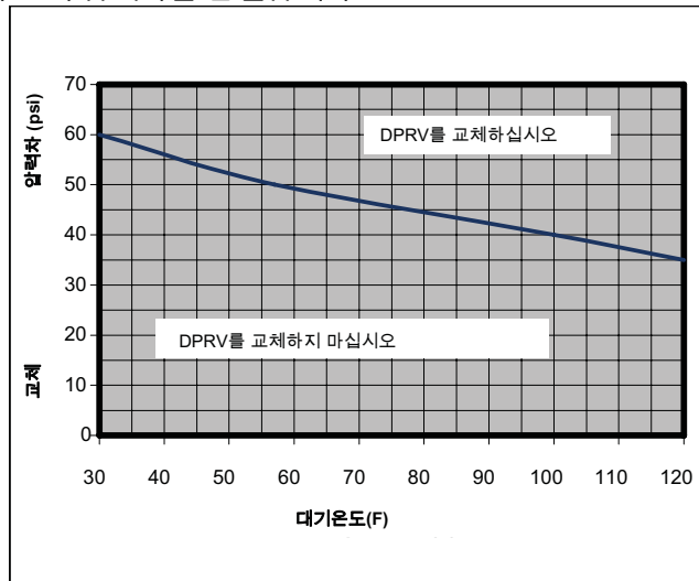
그림 6-25 DPRV 교체 밸브 차트
