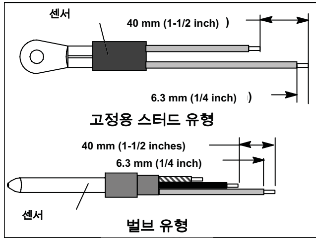
그림 6-27 센서 유형
