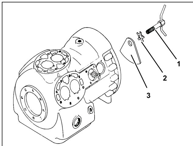
그림 6-12 이퀄라이징 튜브와 잠금 나사 조립체
