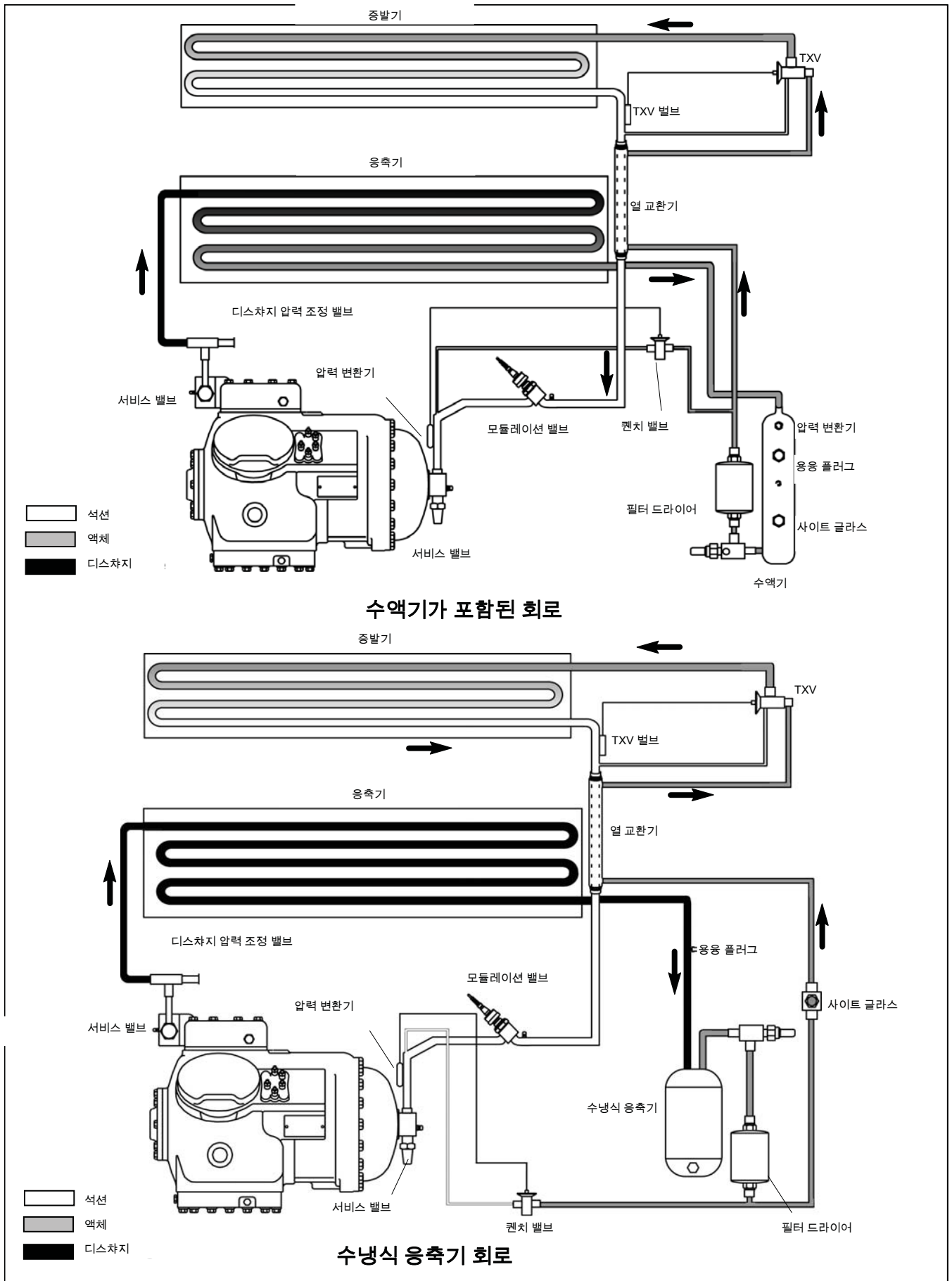
그림 2-7 냉동 회로 구성도
