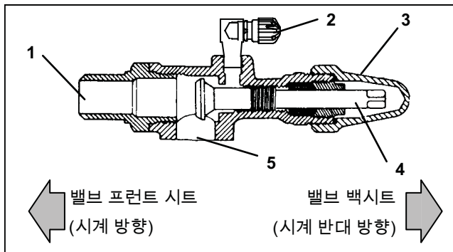
그림 6-1 서비스 밸브
