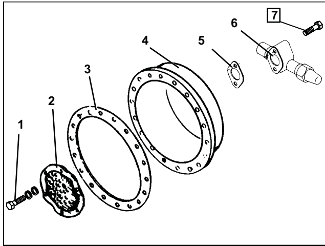
그림 6-11 모터 엔드 커버
