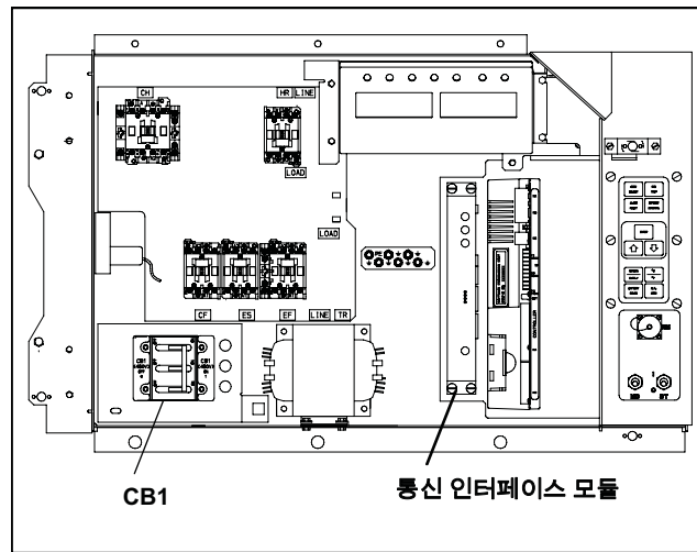
그림 6-34. 통신 인터페이스 설치
