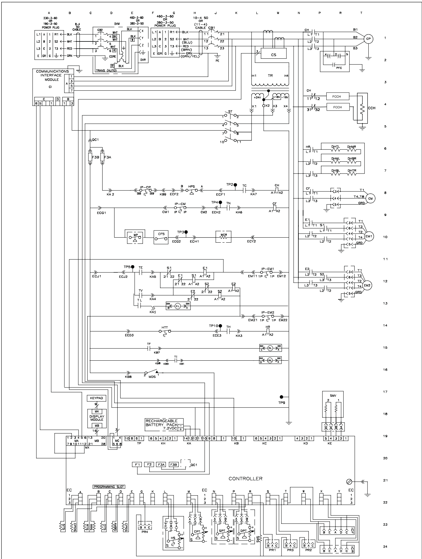
그림 7-3 구성도 - 단일 중발기 팬을 갖춘 유닛
