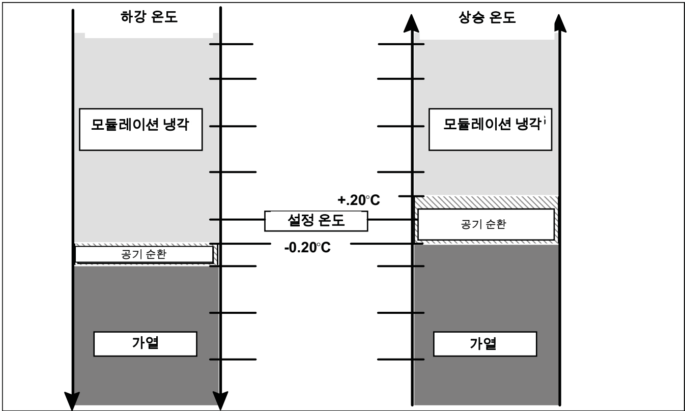
그림 4-3 컨트롤러 작동 - Perishable(냉장) 모드
