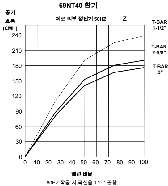
그림 4-2 공기 흐름 차트 작성
