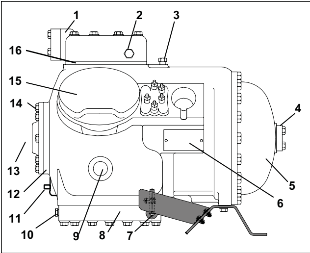
그림 6-6 압축기
