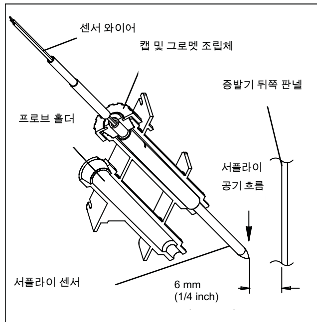
그림 6-29 서플라이 센서 위치
