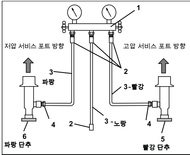
그림 6-3 R-134a 매니폴드 게이지/호스 세트 연결
